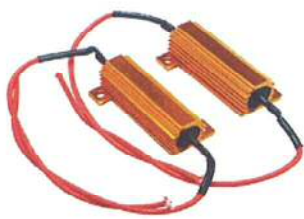
LEDウィンカー用 ハイフラ防止 抵抗ユニット VT-RES27 (2個1SET)
