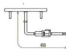
配線寸法
