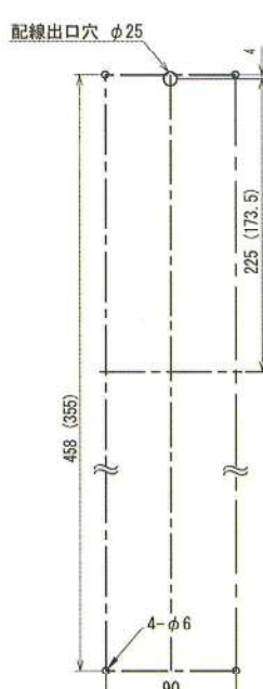
取付寸法
